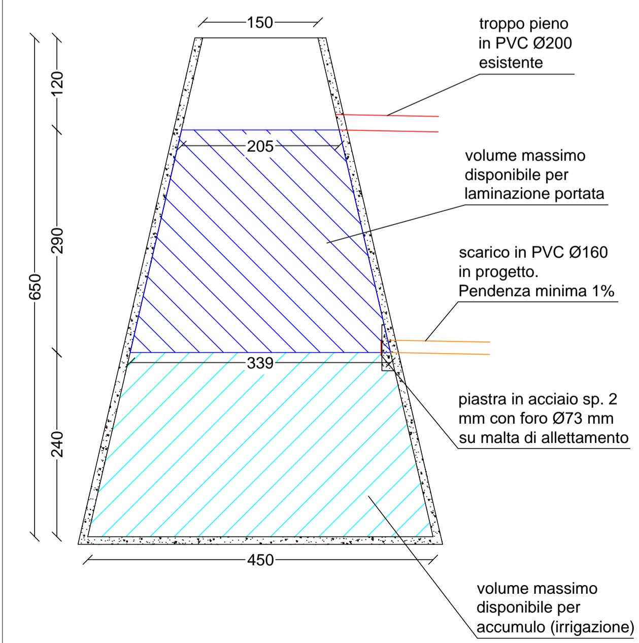
SEZIONE POZZO - scala 1:50
